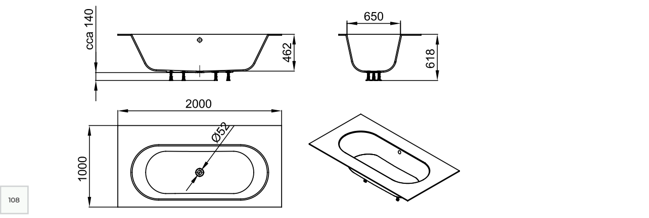
Kerrock bathtub, outflow-overflow set with the UP&DOWN system, installation on tiles or in tile-level, possibility of trimming the edge of the bathtub. Badewanne aus Kerrock, Ab- und Überlaufgarnitur mit UP & DOWN System, Badewanneneinbau auf Bodenfliesen bzw. aufs Bodenfliesen-Niveau, die Badewannenränder können nach Maß zugeschnitten werden. Baignoire en Kerrock. Kit de trop-plein avec système UP&DOWN, pieds de baignoire. Installation sur les plaques ou au niveau des plaques. Possibilité de découper le bord de la baignoire.
