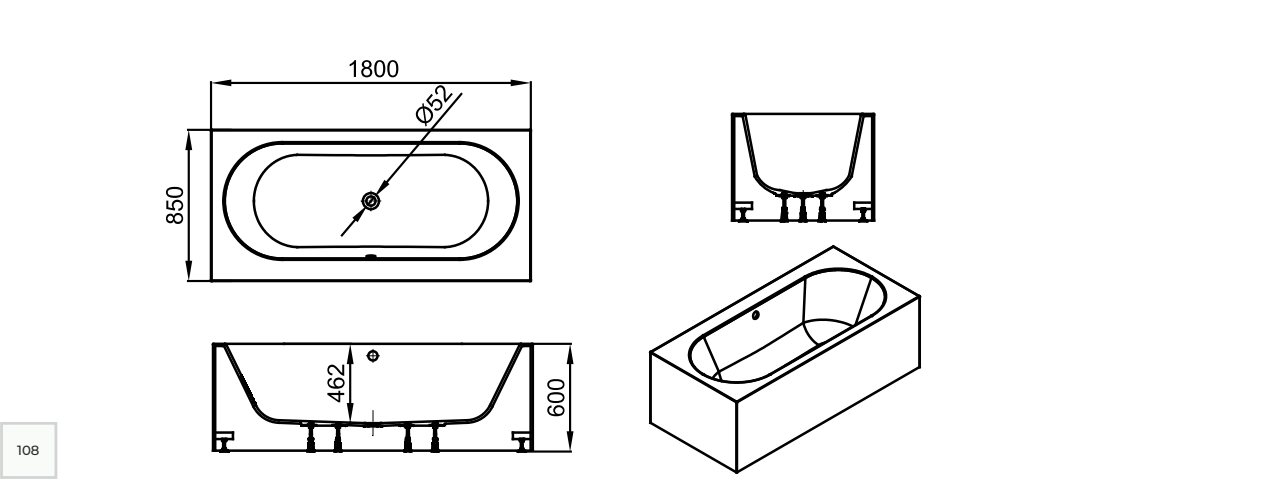
Freestanding Kerrock bathtub, outflow-overflow set with the UP&DOWN system. Freistehende Badewanne aus Kerrock, Ab- und Überlaufgarnitur mit UP & DOWN System. Baignoire autoportante en Kerrock. Kit de trop-plein avec système UP&DOWN.
